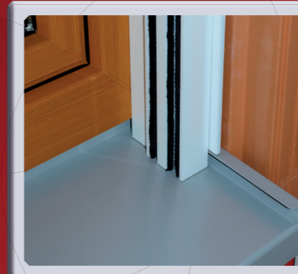
Doppelaufschiene
