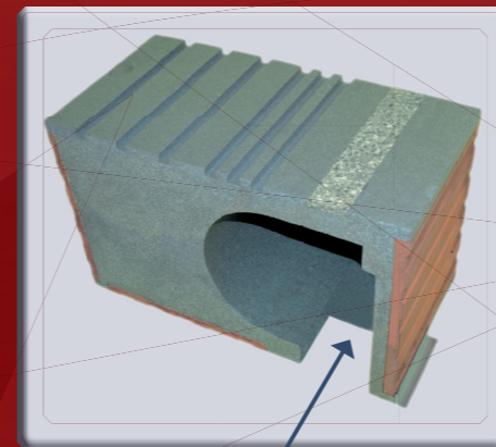
Auflagerdämmung mit oben- liegender Behangshalterung
