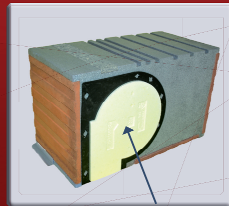
hochdämmende, seitliche Kopfstückisolierung
