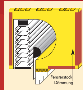
Raffstore mit integriertem Fliegengitter-Rollo
