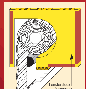
Jalousiesystem mit Zusatzisolierung
