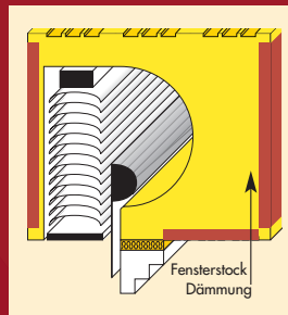
Jalousiesystem mit integriertem Fliegengitter-Rollo
