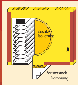
Raffstore mit Zusatzisolierung
